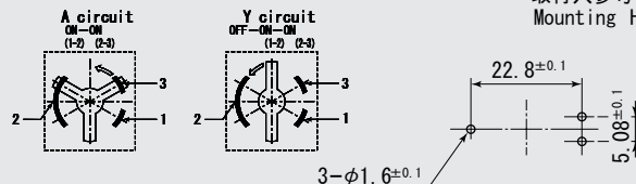
取付穴参考寸法 Mounting Hole
